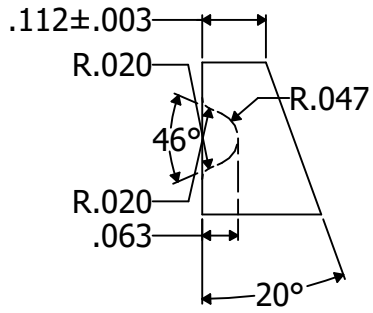
14WMP-1 1/2" GASKET GROOVE DETAIL
